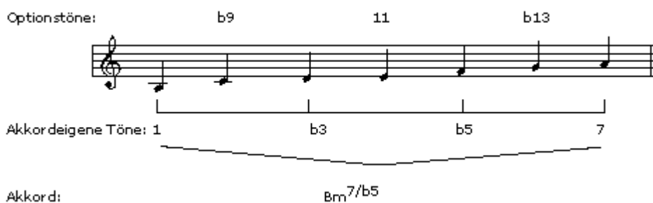
Abb.58 Lokrische Skala:
