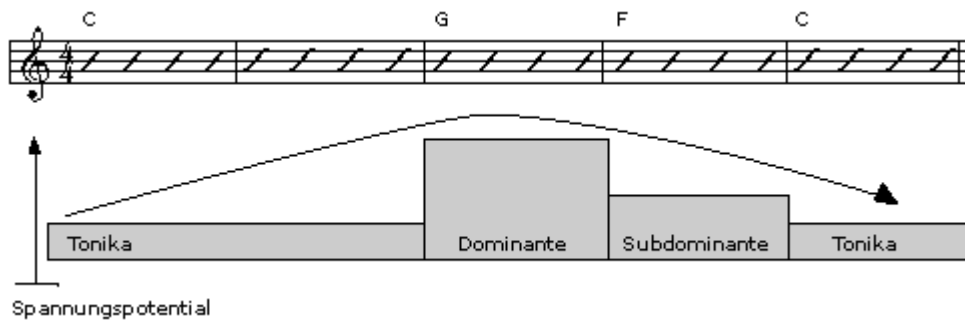
Abb.8 Plagale Kadenz
