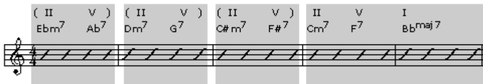
Abb.25 II-V- Verkettungen
