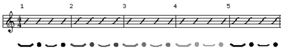
Abb. 69 Metrisches Spannungsmodell:
